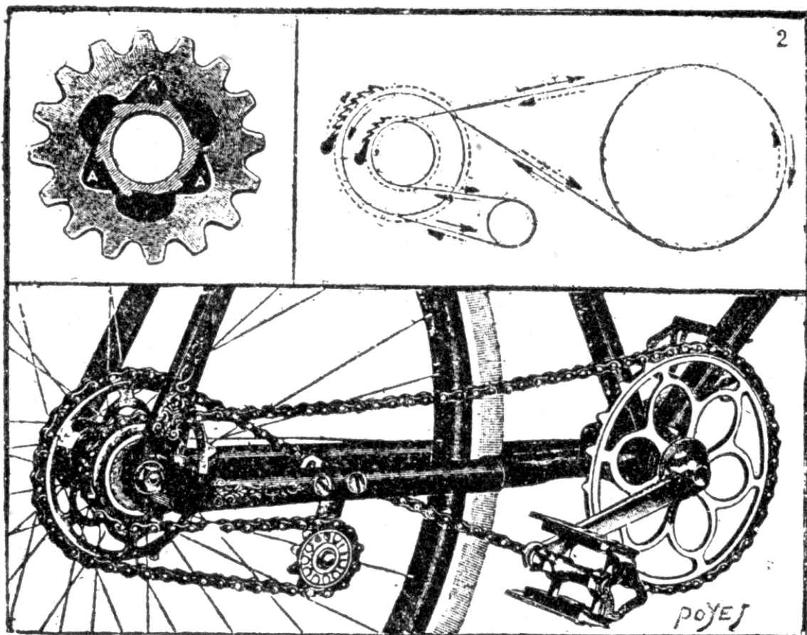
Převod jízdního kola se dvěma rychlostmi.
